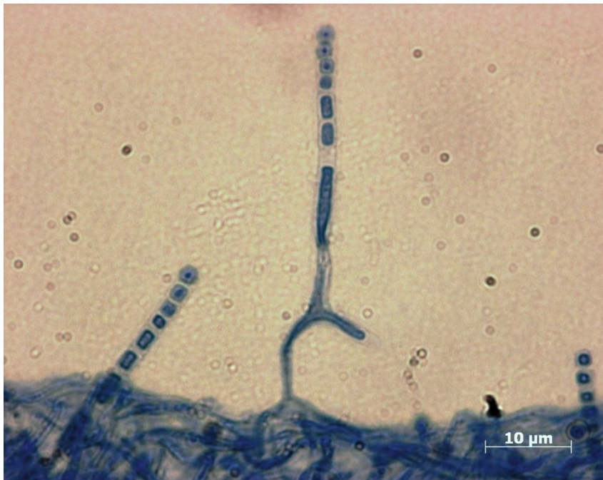
Wallemia-4
