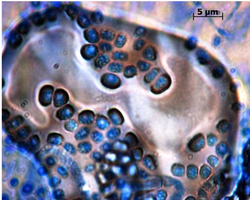
Wallemia-7
