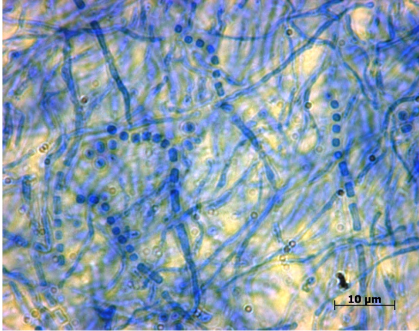
Wallemia-6
