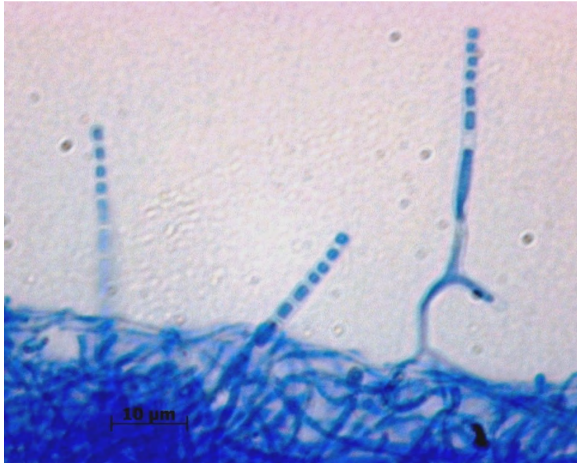
Wallemia-3
